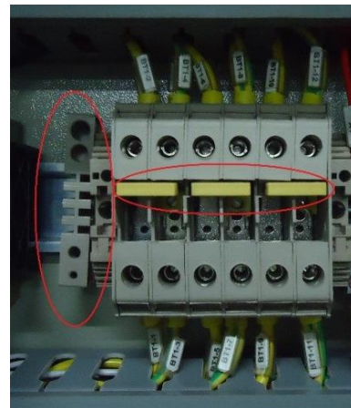
Fig.2: Incorreto (Jumper no Bloco)
